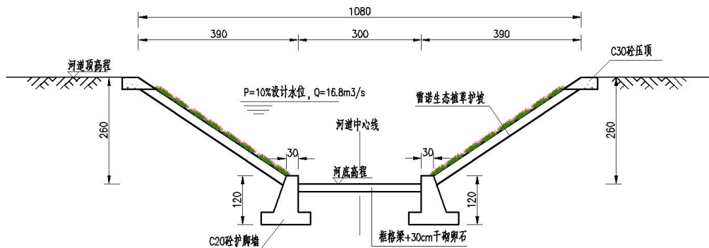
图 1.1-3 渠道工程标准横断面图
