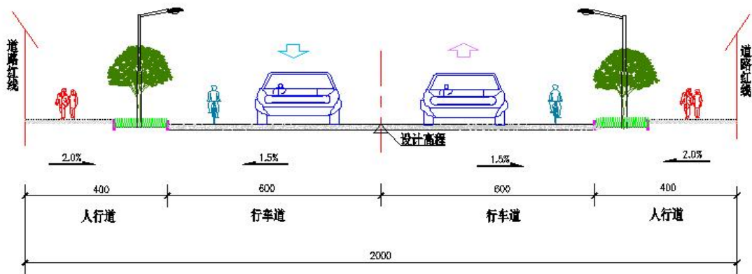
图 1.1-2 路基标准横断面图
